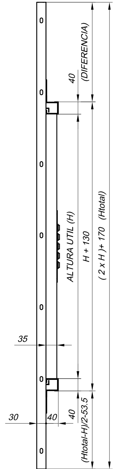
DIMENSIONES DE MONTAJE
